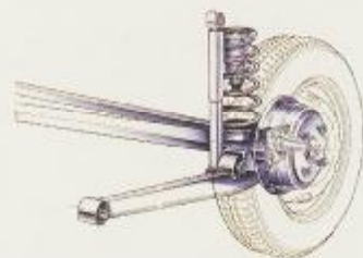
Zadná tuhá náprava s pozdĺžnymi vodiacími ramenami
